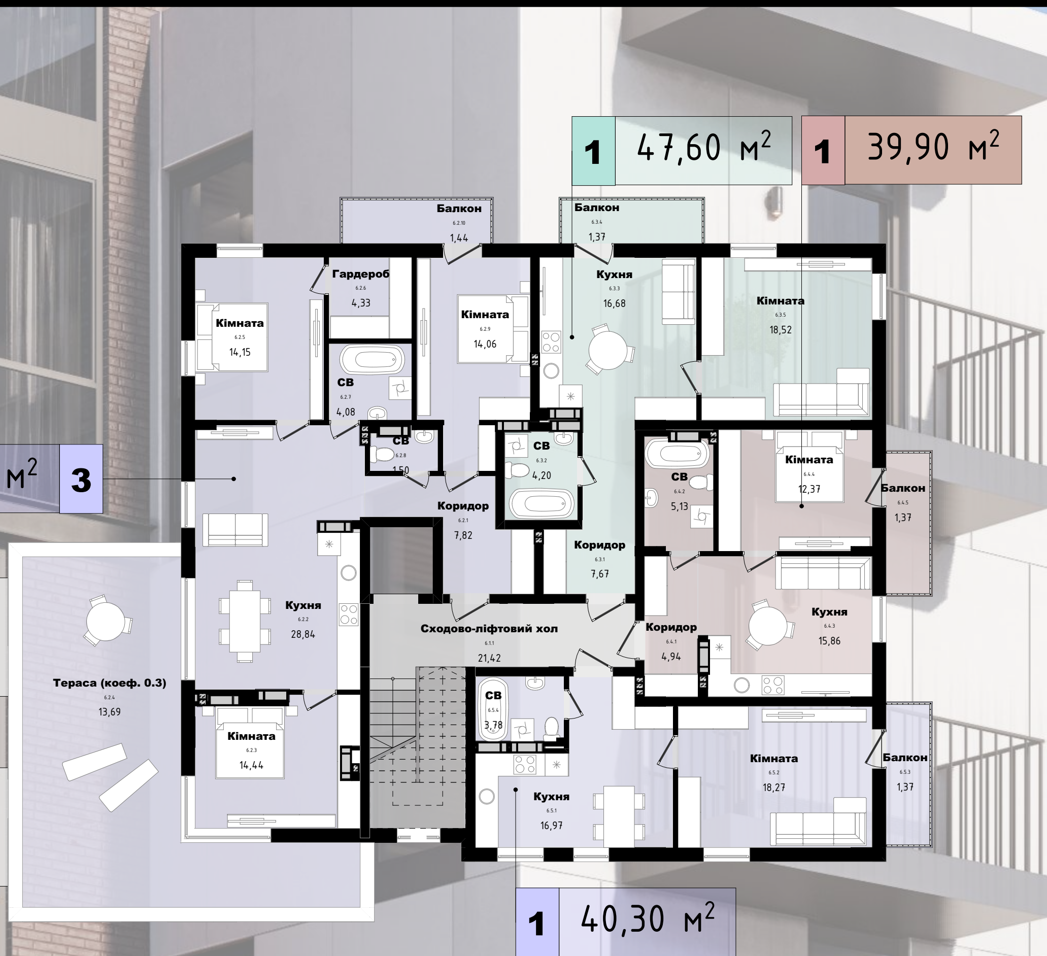
План 6-го поверху
